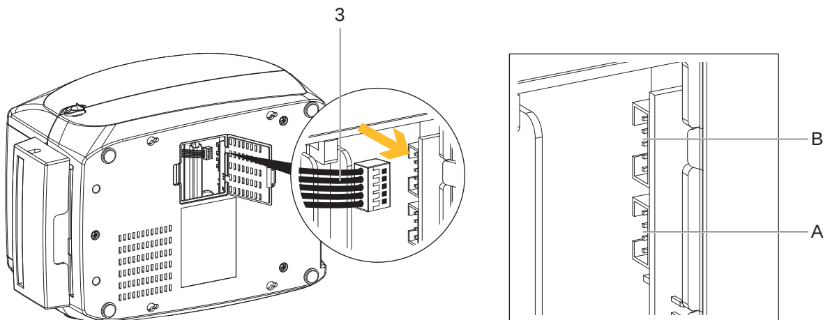
Bild 40 Verbindungskabel anschließen
