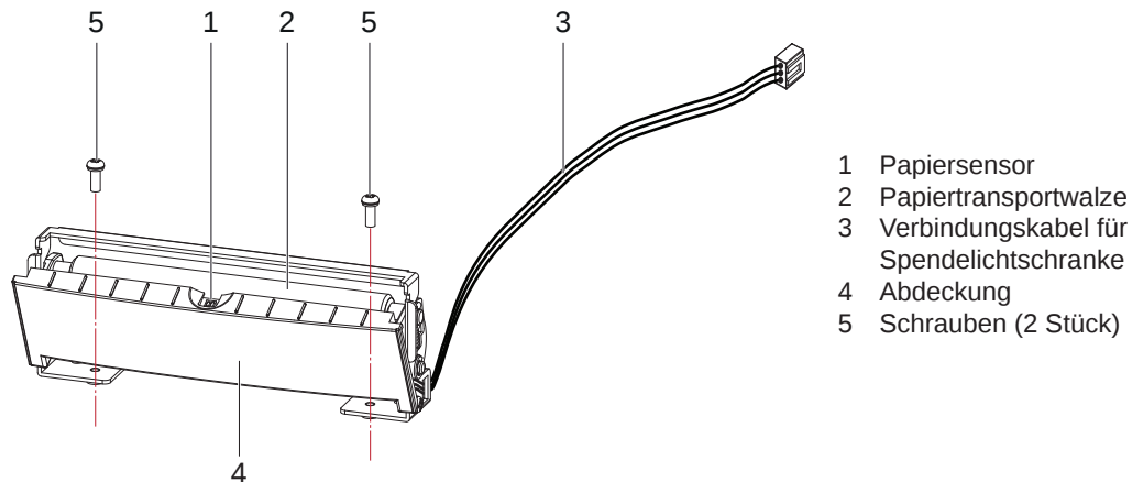
Bild 25 Geräteübersicht Spendellichtschränke
