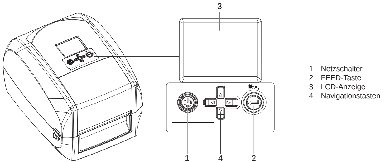
Bild 19 Übersicht Bedienfeld
