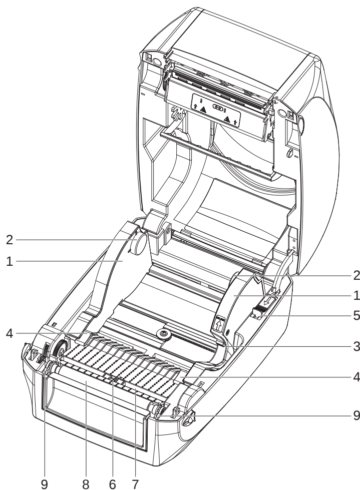
Bild 5 Innenansicht
