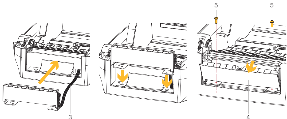
Bild 26 Spendellichtschränke montieren
