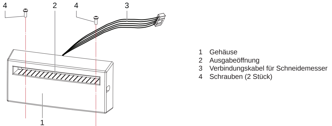
Bild 35 Geräteübersicht Schneidemesser
