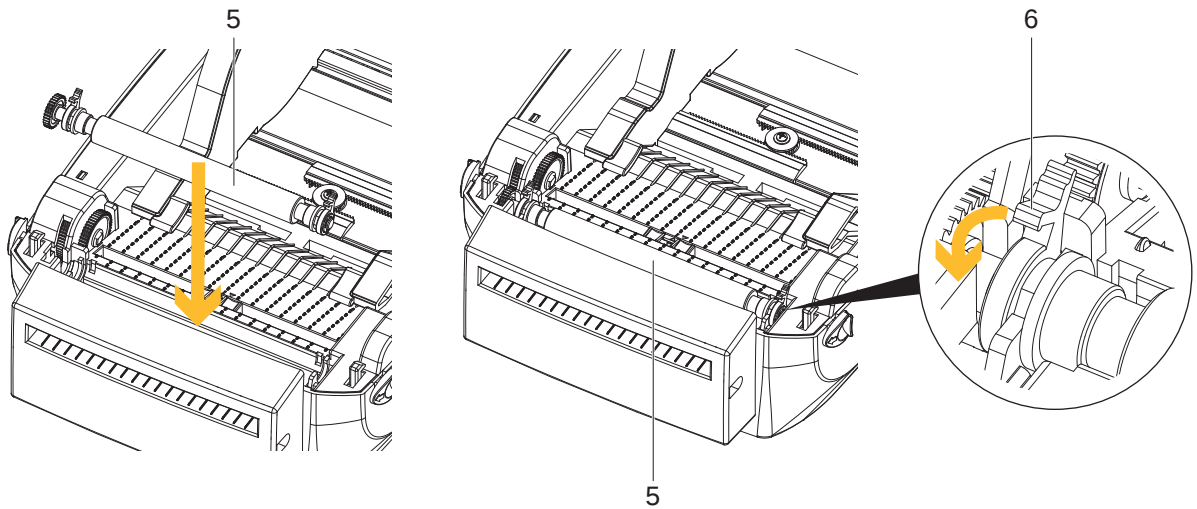
Bild 37 Druckwalze einsetzen
