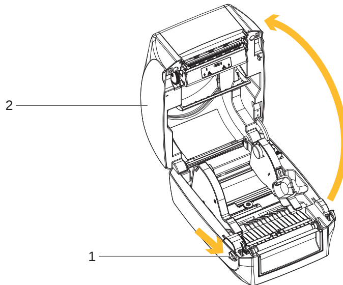
Bild 22 Drucker öffnen
