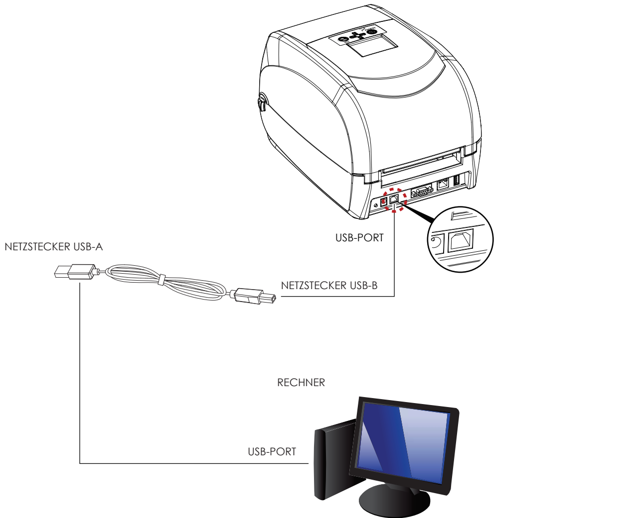
RT700i/RT730i BARCODE-DRUCKER
